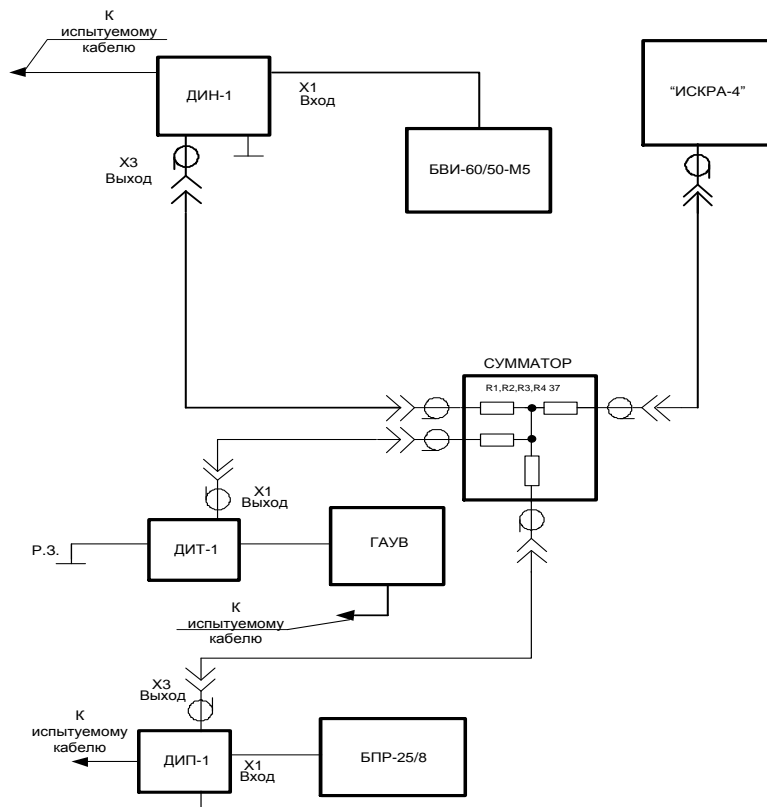
Рис. 10б. Подключение прибора «Искра 4» в электролаборатории с датчиком ДИН-1, ДИП-1 и ДИТ-1
