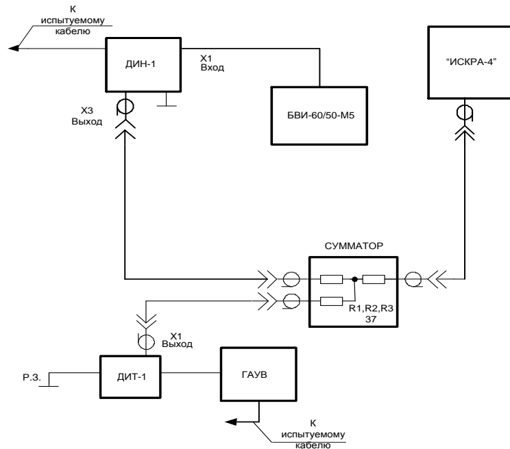
Рис. 10а. Подключение прибора «ИСКРА-4» в электролаборатории с датчиками ДИТ-1 и ДИН-1
