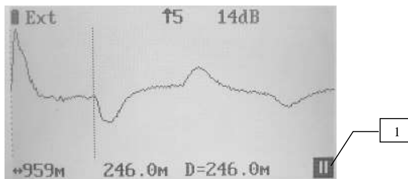
Рис. 30а. Пример рефлектограммы места повреждения в режиме работы «Испытание»/«Прожиг» (метод Desau)
